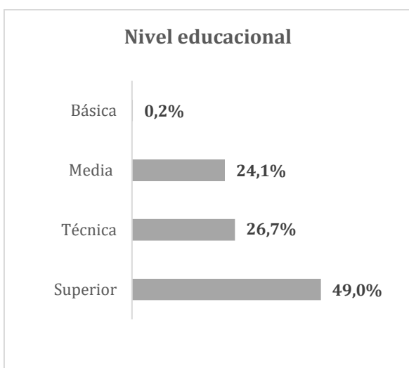
Gráfico 3: Nivel educacional
